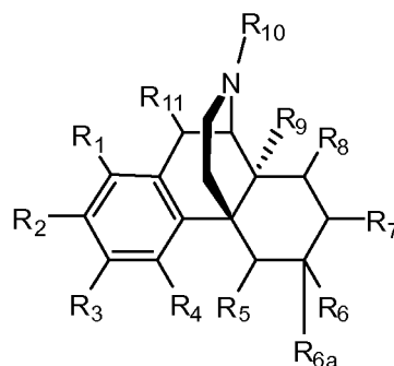
Formula I(d)
