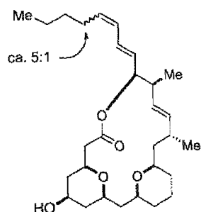
Analog 4 (HF27164)
