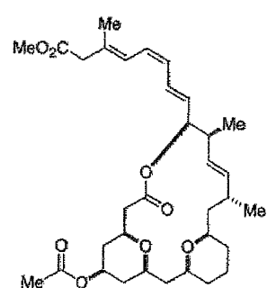
Analog 2 (HF27156)
