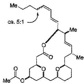
Analog 3 (HF27162)
