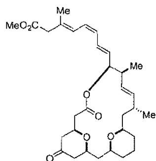
Analog 7 (HF27187)
