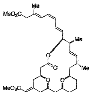
Exiguolide (HF26074)
