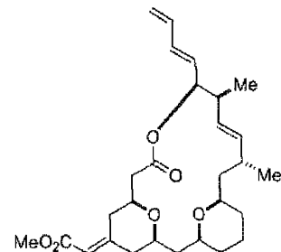
Analog 6 (HF27192)
