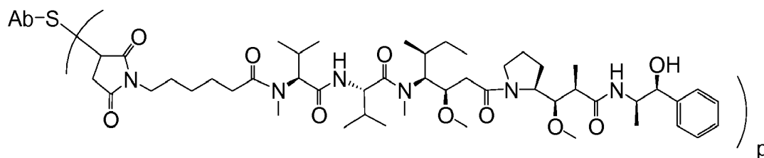
Ab-MC-vc-PAB-MMAE
