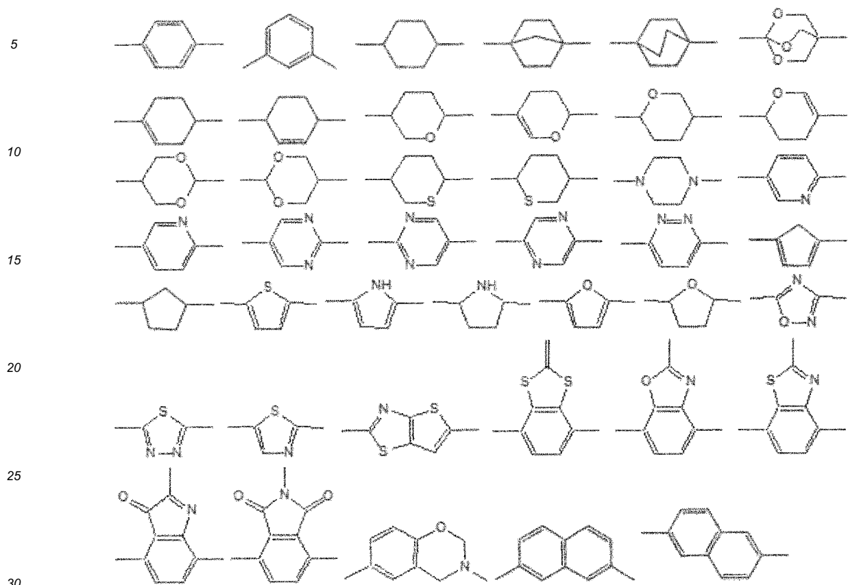
[Chem. 5]
