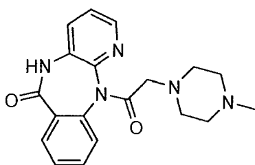
Pirenzepine
