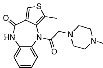
Telenzepine
