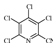
17% Cl 4 -PN
