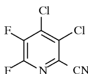
2.3% 5,6-F 2 -PN
