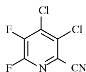
2.3% 5,6-F 2 -PN
