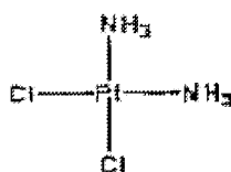
cisplatin cis-DDP
