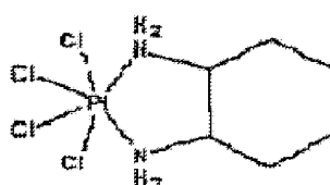
ormaplatin letraplatin
