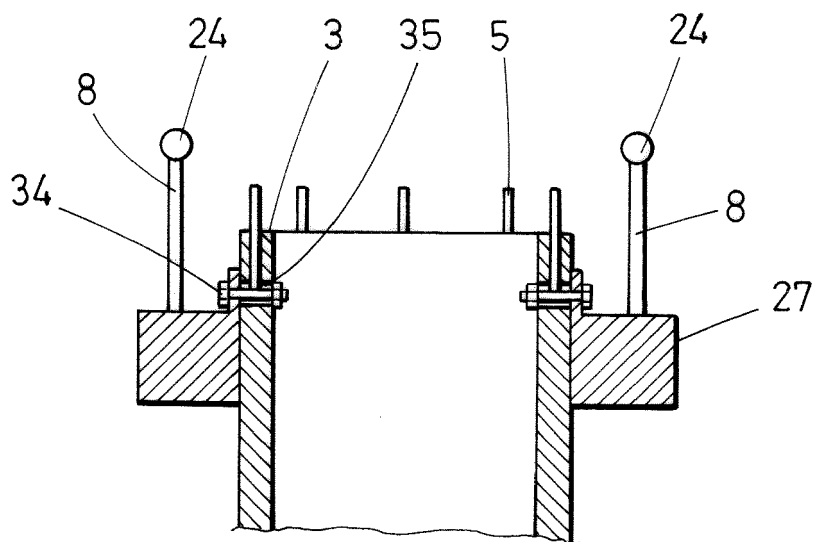
A-A' FIG.11
