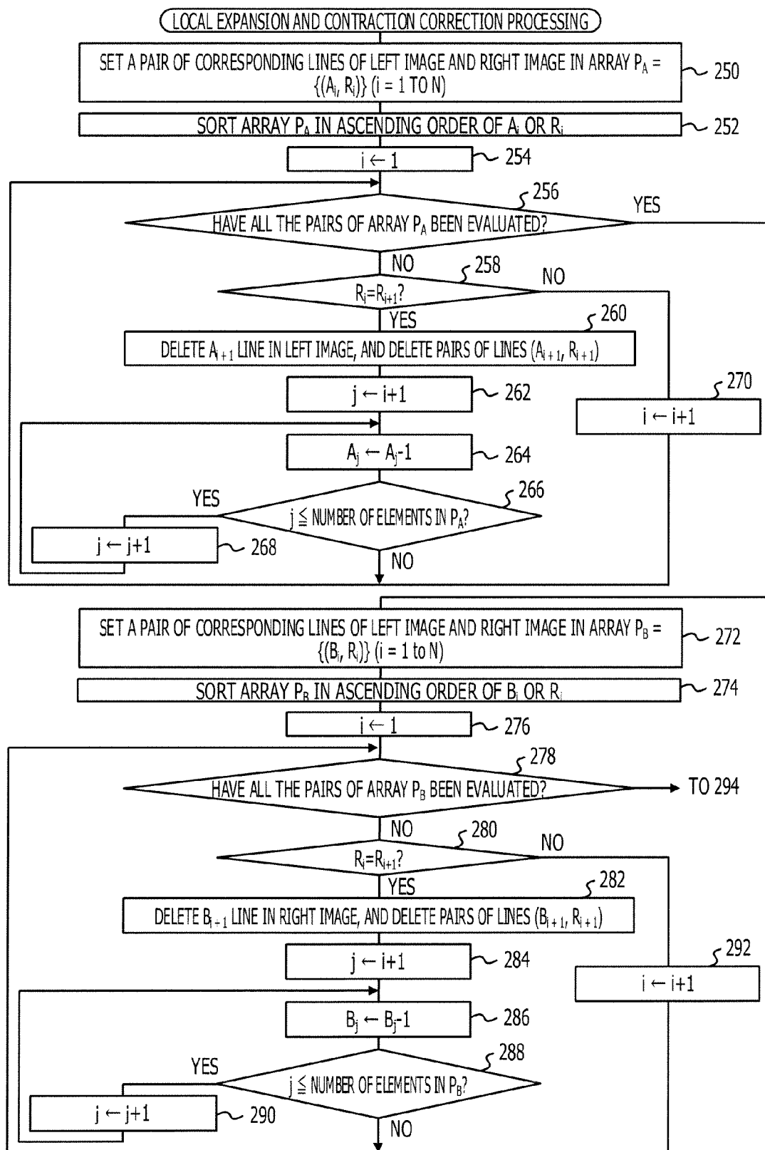
FIG. 24A
