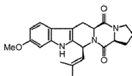
Fumitremorgin C
