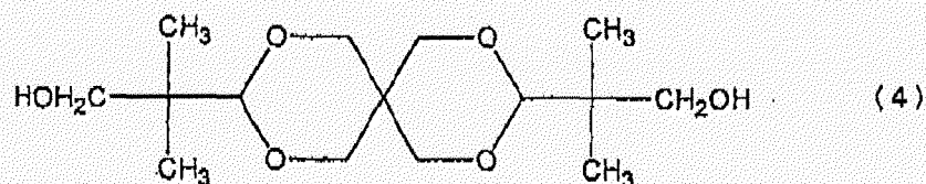
[Chem. 6]
