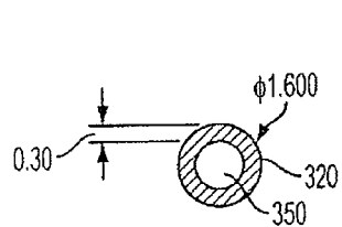
SECTION A-A SCALE 16.000
