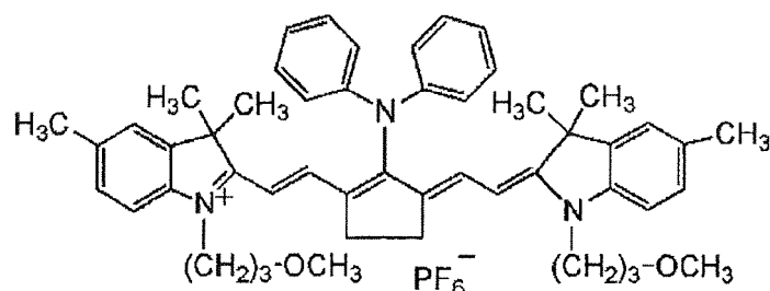
IR absorber (1)
