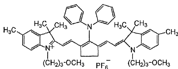
IR absorber (1)
