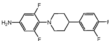
(4-(4-(3,4-difluorophenyl)piperidin-1-yl)-3,5-difluoroaniline)
