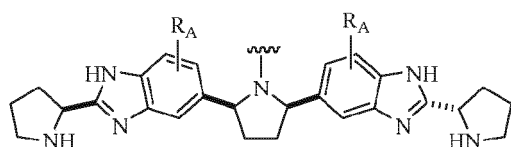
11-1
