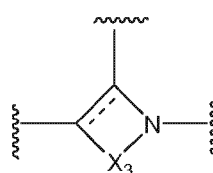
X-3
