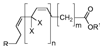
11,11,14,14-Tetramethyl-octadeca-9,12,15-trienoic acid
