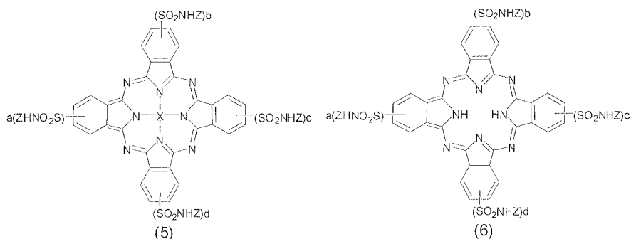
[Chem. 3]
