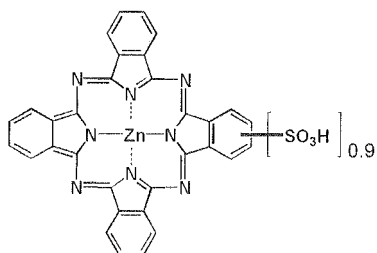
[Chem. 5]
