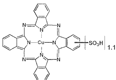
[Chem. 6]
