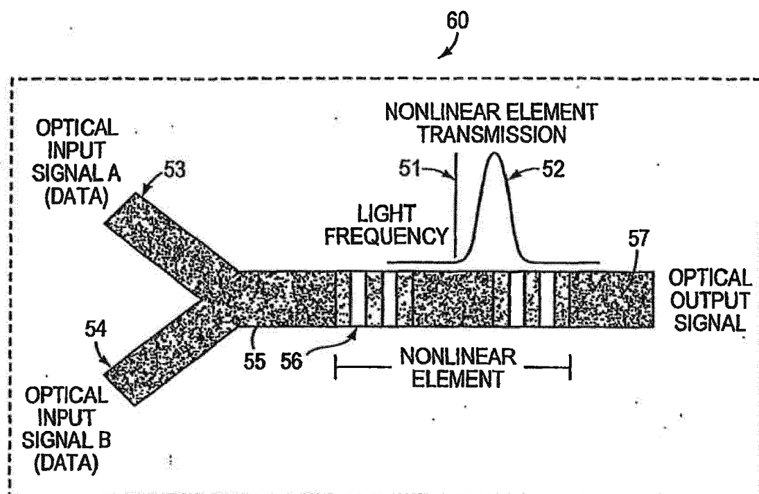
ALL-OPTICAL XOR GATE
