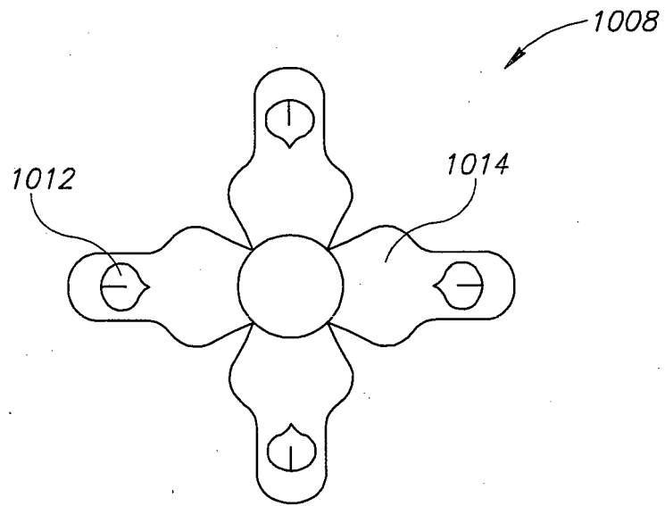
FIG.10C VIEW A-A
