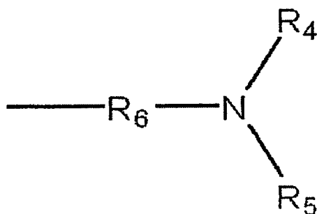
Formule structurale (3)
