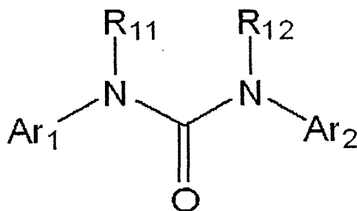
Formule structurale (4)
