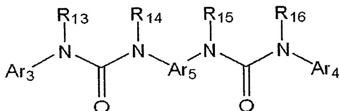
Formule structurale (5)
