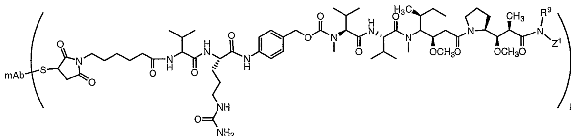
Ab-MC-vc-PAB-MMAZ
