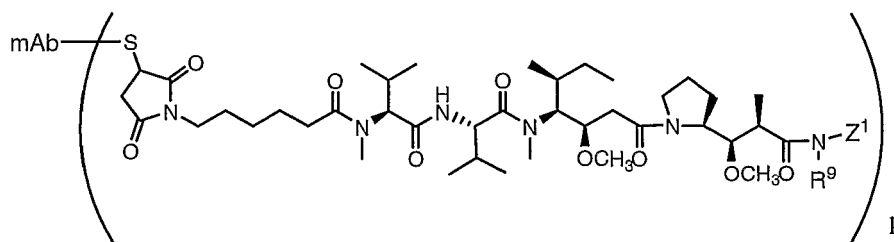
Ab-MC-MMAZ
