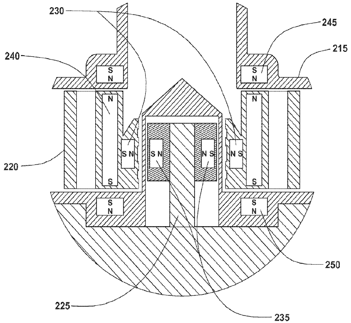
FIG. 20 (DETAIL H)
