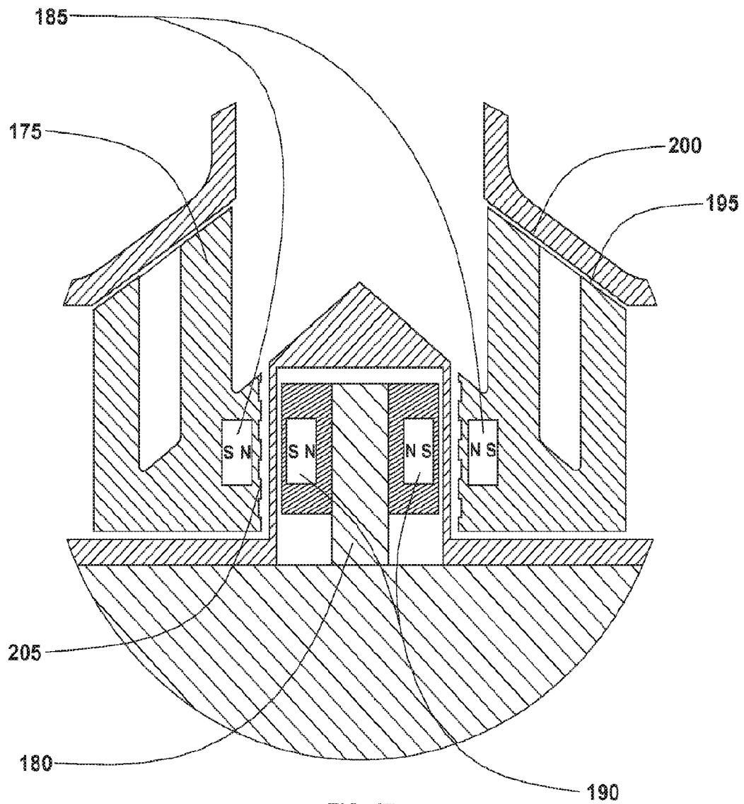
FIG. 17 (DETAIL E)
