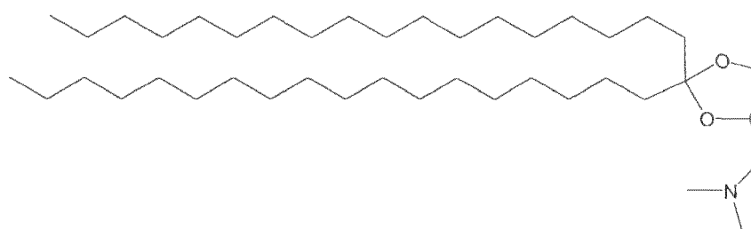
DS-K-DMA;
