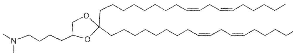
DLin-K-C4-DMA.
