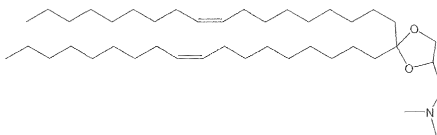
DO-K-DMA;
