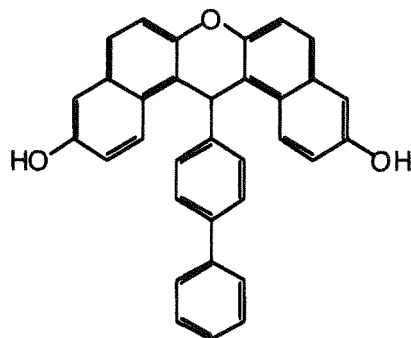
(XBisN-1)
