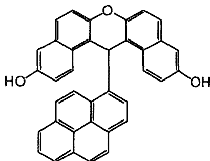
(XBisN-9)
