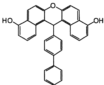
(XBisN-4)
