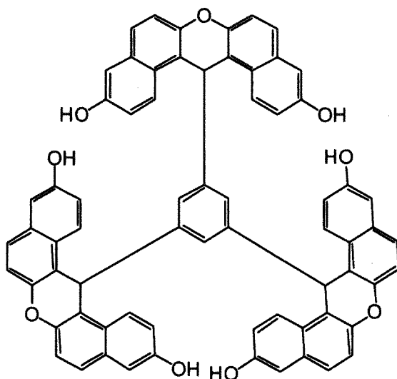
(XBisN-14)
