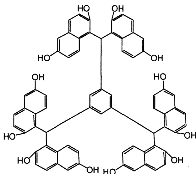
(XBisN-1)
