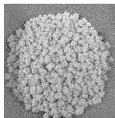
MIL-125(Ti)_NH 2 Composite
