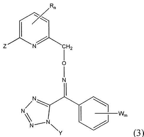
[Chem. 3]
