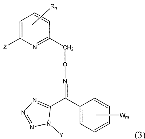
[Chem. 3]
