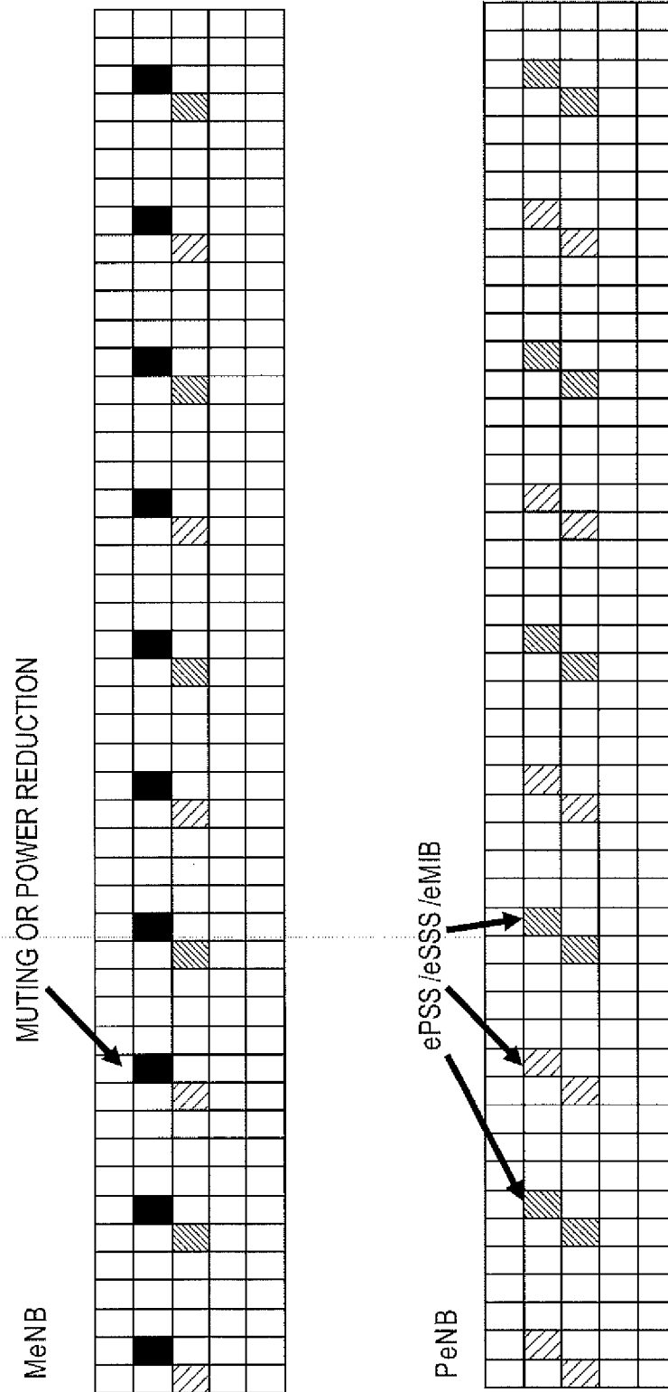
FIG. 9 ePSS/eSSS/eMIB SUBFRAME SYNC.
