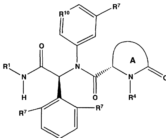
Formel II-a
