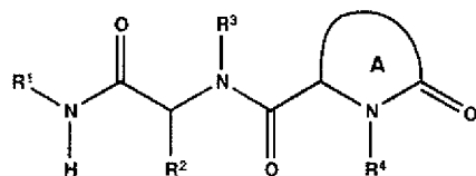
formule I
