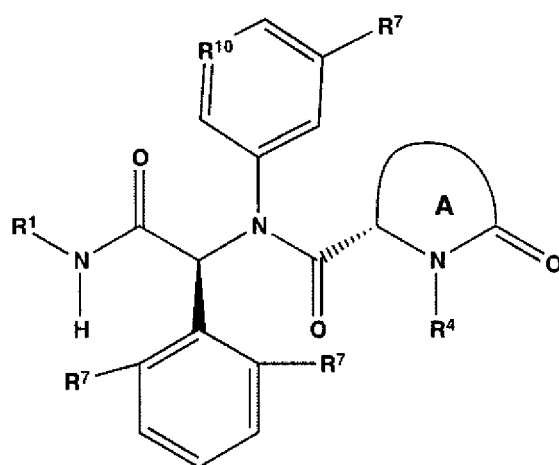
formule II-a
