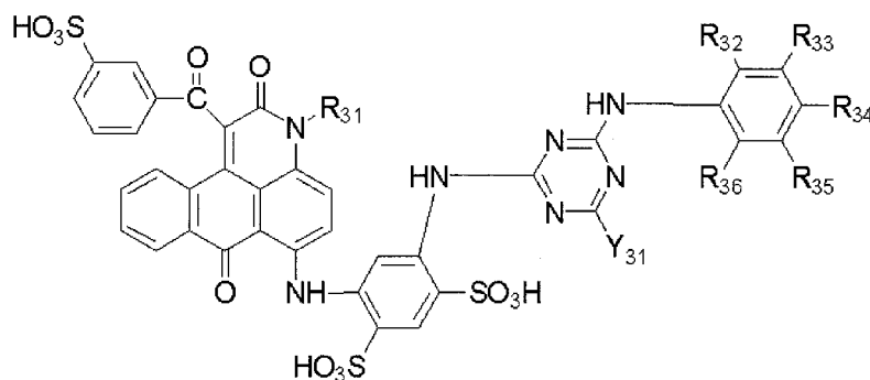
(B 5 - 5)
