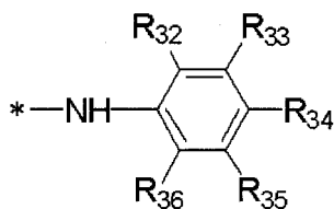
( B 5 - 1 )
