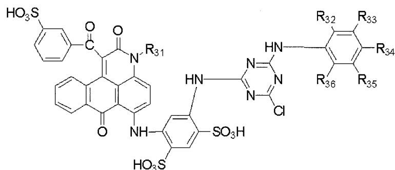
(B 5 - 4)
