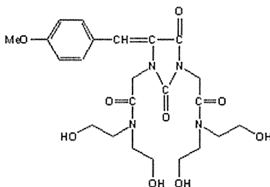
5-(4-methoxybenzylidenel-1,3-bis[2-[bis(2-hydroxyethyl)amino]-2-oxoethyl]hydantoin
