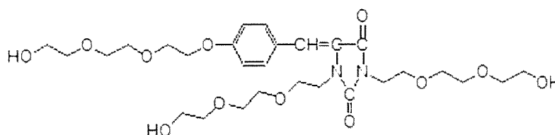
5-[4-[2-[2-(2-hydroxyethoxy)ethoxy]ethoxy]benzylidene]-1,3-bis[2-[2-(2-hydroxyethoxy)ethoxy]ethyl]hydantoin
