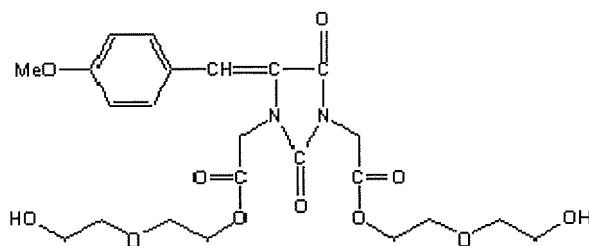
5-(4-methoxybenzylidene)-1,3-bis[2-[2-(2-hydroxyethoxy)ethoxy]-2-oxoethyl]hydantoin
