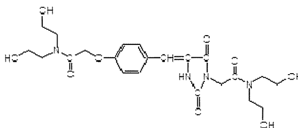
5-[4-[2-[bis(2-hydroxyethyl)amino]-2-oxoethoxy]benzylidene]-3-[2-[bis(2-hydroxyethyl)amino]-2-oxoethyl]hydantoin
