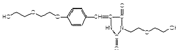
5-[4-[2-(2-hydroxyethoxy)ethoxy]benzylidene]-3-[2-(2-hydroxyethoxy)ethyl]hydantoin
