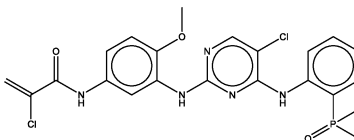
2-chloro- N -(3-((5-chloro-4-((2-(dimethylphosphoryl)phenyl)amino)pyrimidin-2-yl)amino)-4-methoxyphenyl)acrylamide
