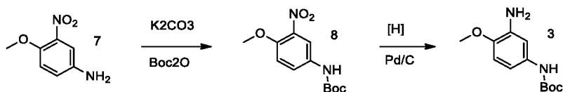
Scheme 1a
