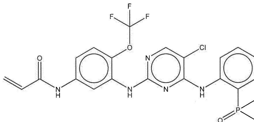
N -(3-((5-chloro-4-((2-(dimethylphosphoryl)phenyl)amino)pyrimidin-2-yl)amino)-4-(trifluoromethoxy)phenyl)acrylamide
