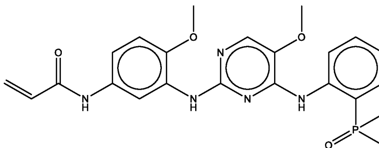
N -(3-((4-((2-(dimethylphosphoryl)phenyl)amino)-5-methoxypyrimidin-2-yl)amino)-4-methoxyphenyl)acrylamide
