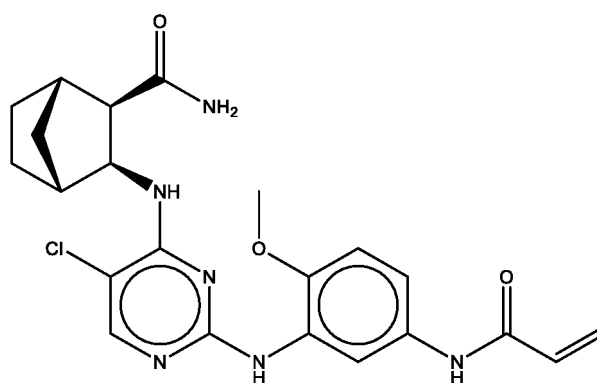
(1 S ,2 R ,3 S ,4 R )-3-((2-((5-acrylamido-2-methoxyphenyl)amino)-5-chloropyrimidin-4-yl)amino)bicyclo[2.2.1]heptane-2-carboxamide
