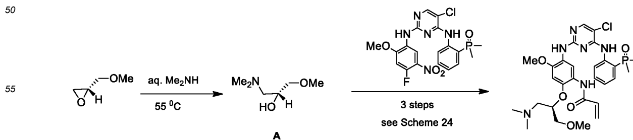
Scheme 43:
