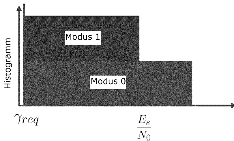
Fig.4 Histogramm von E_s/N_0 für eine Multi-Modus-Einstellung
