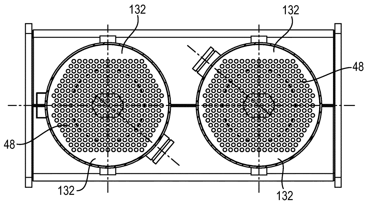
FIG. 9C
