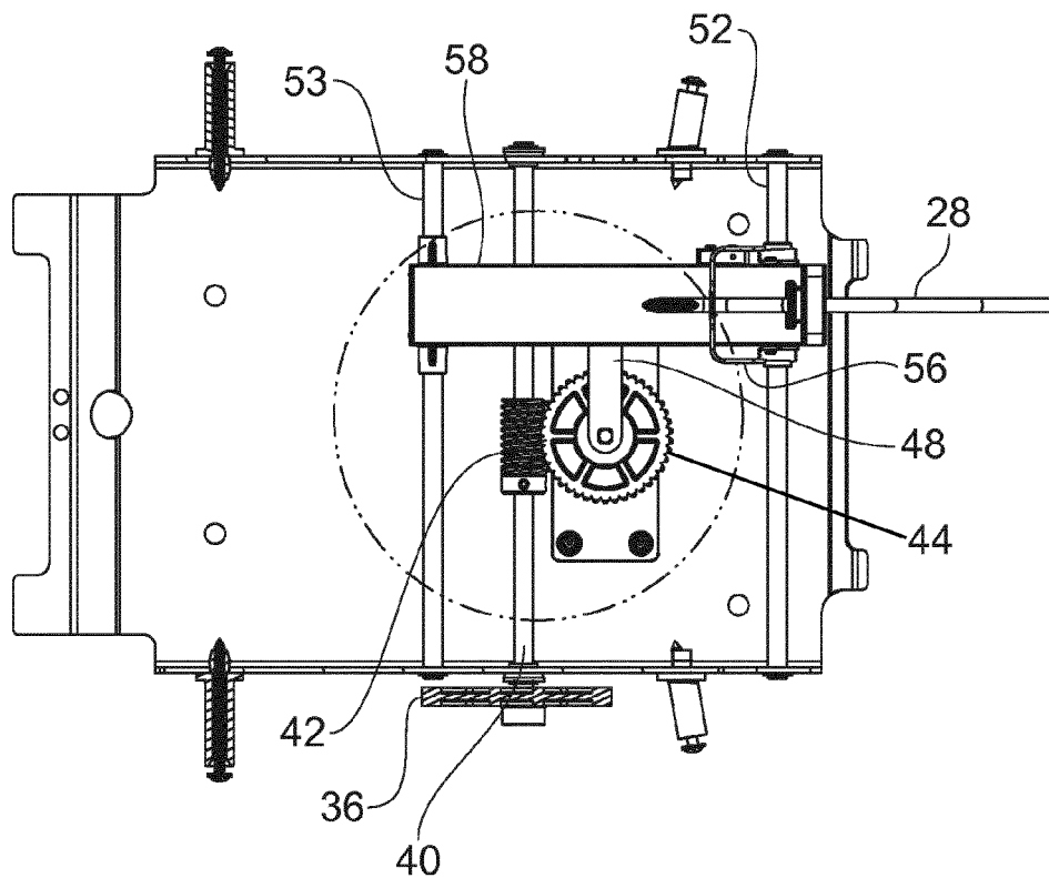
FIG. 4 SECTION V-V
