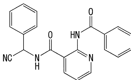
[Chem. 3]
