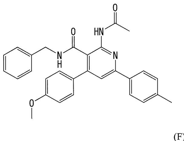
[Chem. 6]
