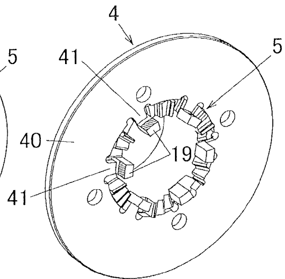
FIG. 9D
