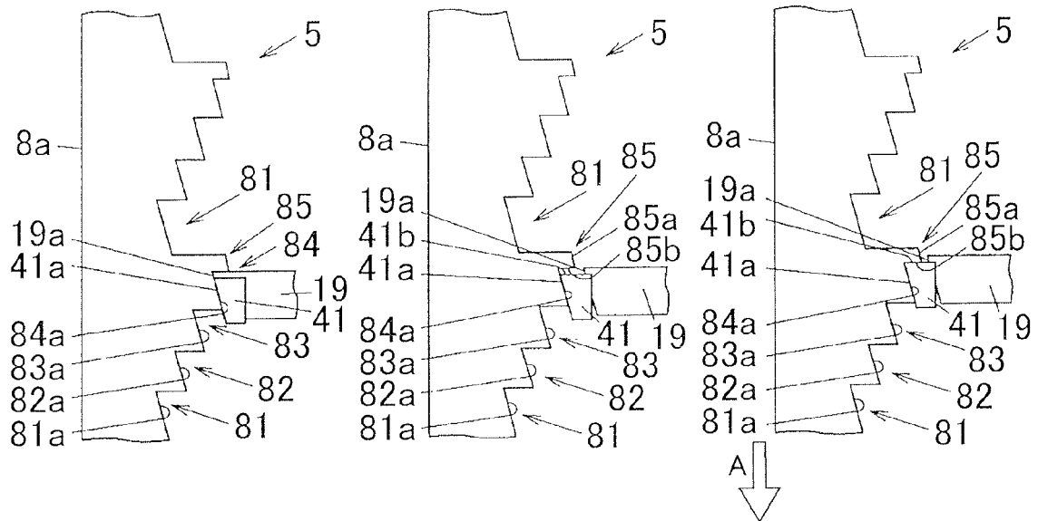
FIG. 10E
