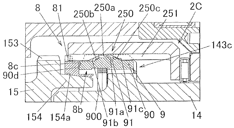
FIG. 24C
