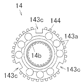
FIG. 21C
