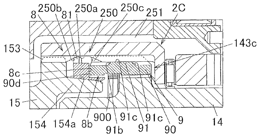
FIG. 24C
