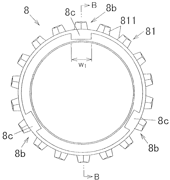
FIG. 22C
