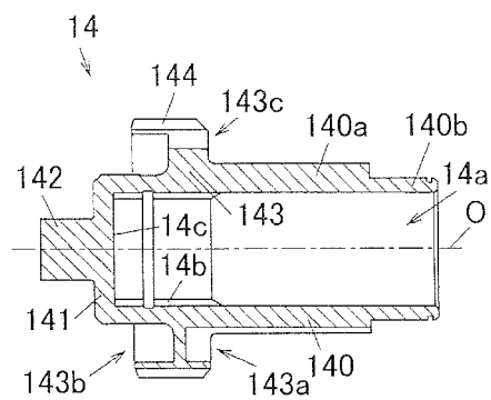
FIG. 21B
