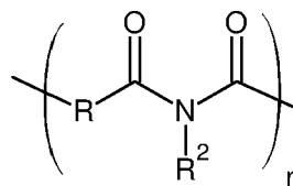
linear polyimide
