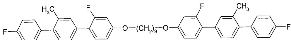
F-PPI(1)GI-O9O-GP(1)P-F
