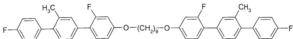
F-PPI(1)GI-O9O-GP(1)P-F
