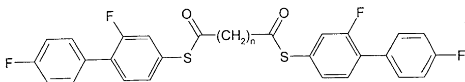
F-PGI-SConCOS-GP-F
