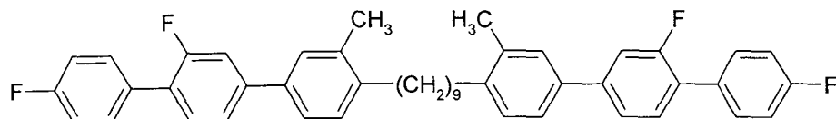
F-PGIP(1)-9-PI(1)GP-F
