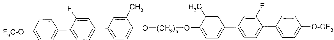
N-PGIP(1)-OnO-PI(1)GP-N
