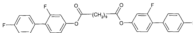
F-PGI-ZI9Z-GP-F
