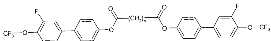
TO-GIP-ZInZ-PG-OT
