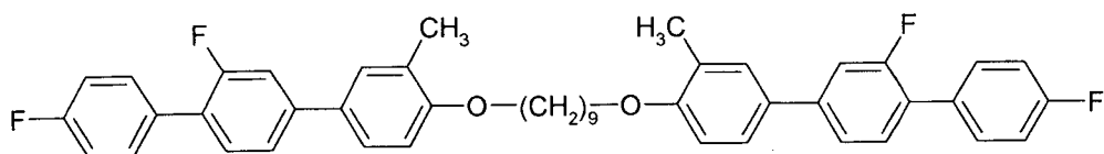
F-PGIP(1)-O9O-PI(1)GP-F
