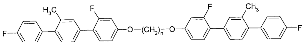
N-PPI(1)GI-OnO-GP(1)P-N
