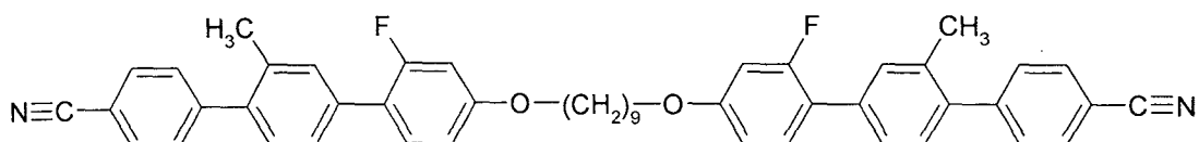
N-PPI(1)GI-O9O-GP(1)P-N
