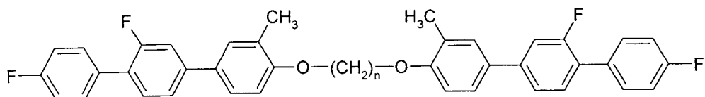
F-PGIP(1)-OnO-PI(1)GP-F
