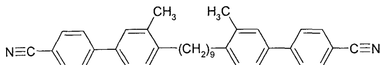
N-PP(1)-9-PI(1)P-N
