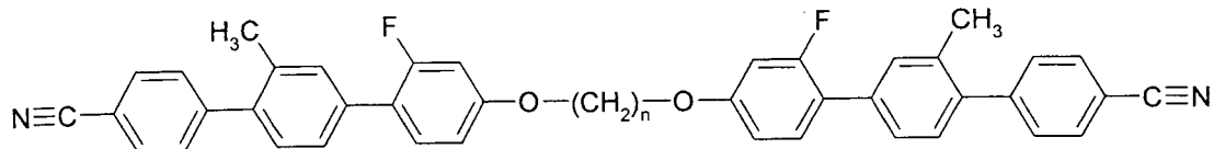
N-PPI(1)GI-OnO-GP(1)P-N
