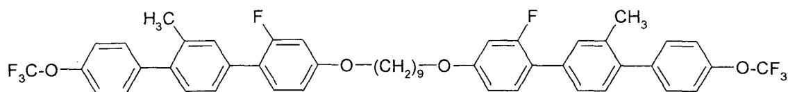
TO-PPI(1)GI-O9O-GP(1)P-OT
