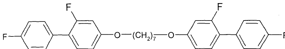
F-PGI-O9O-GP-F
