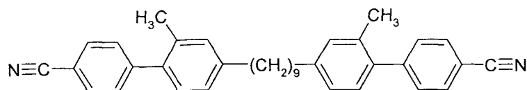
N-PPI(1)-9-P(1)P-N
