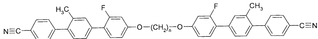
N-PPI(1)GI-OnO-GP(1)P-N
