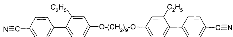
N-PPI(2)-O9O-P(2)P-N
