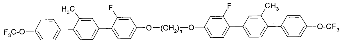
TO-PPI(1)GI-OnO-GP(1)P-OT
