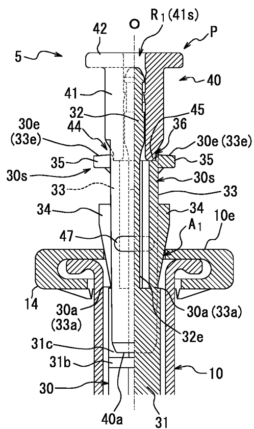
FIG. 14A
