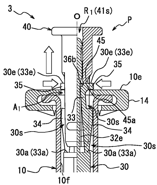
FIG. 10C
