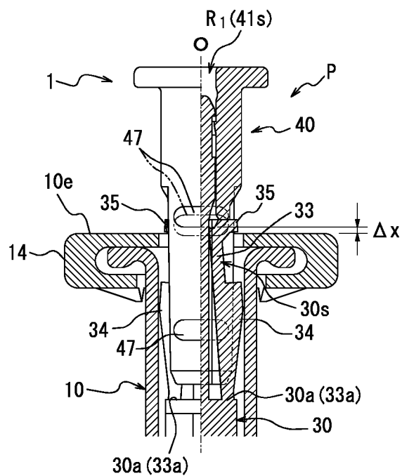
FIG. 12B
