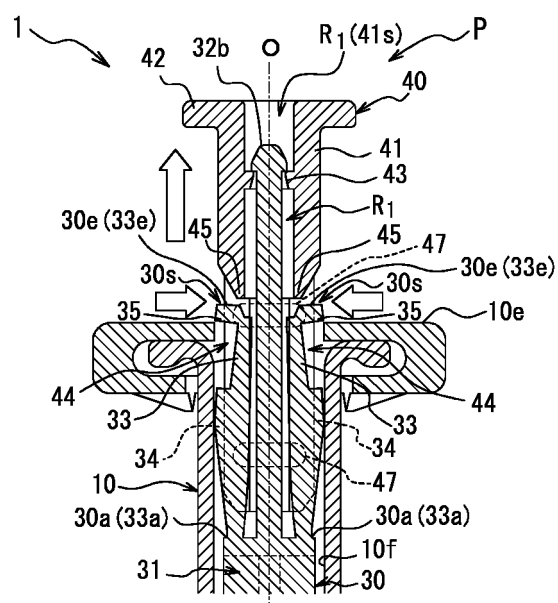
FIG. 3C
