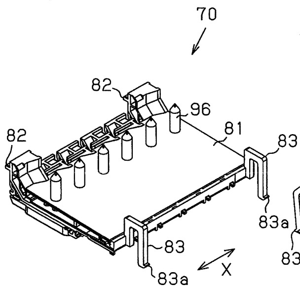
Fig.19A
