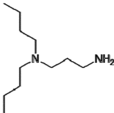
N,N'-dibutylpropane-1,3-diamine
