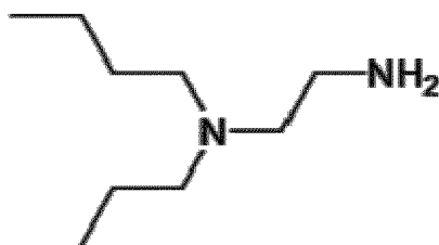
N 1 ,N 1 -dibutylethane-1,2-diamine
