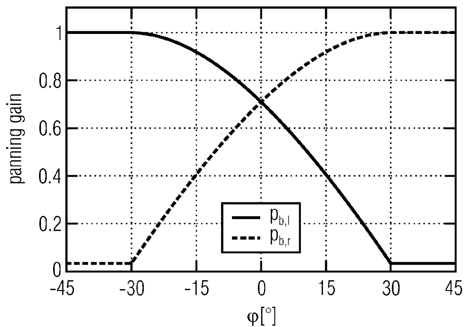
VBAF panning function
