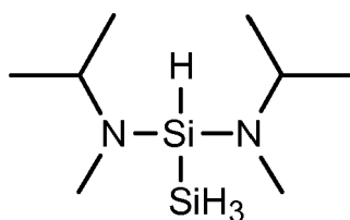
1,1-bis(isopropylmethylamino)disilane
