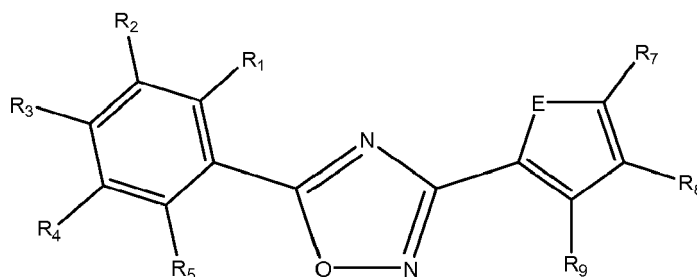
Formula Va
