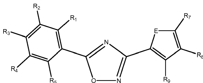
Formula Va
