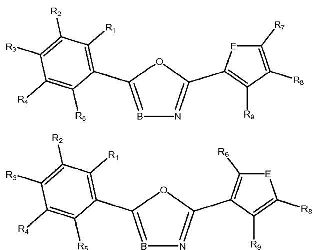
Formulas:
