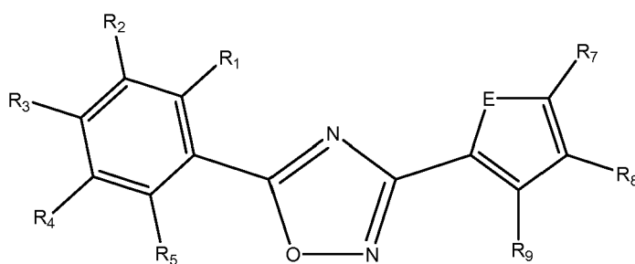
Formula Va
