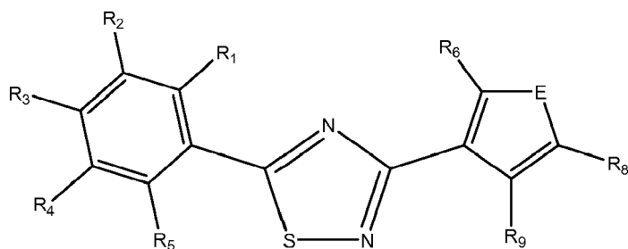
Formula VIIb
