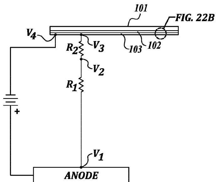
FIG. 22A
