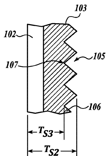
FIG. 22C
