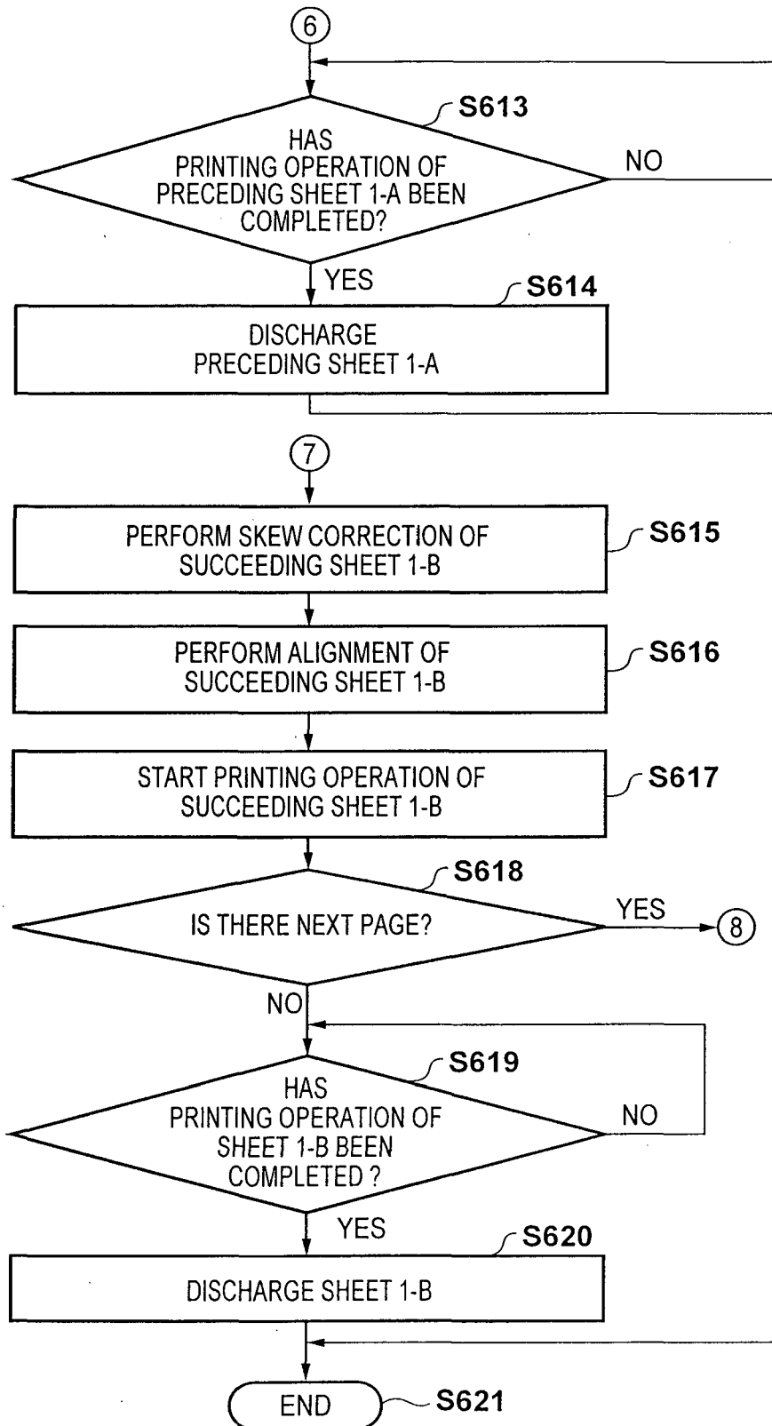
FIG. 15B
