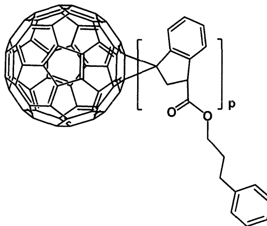
[Formula 1-1-44]
