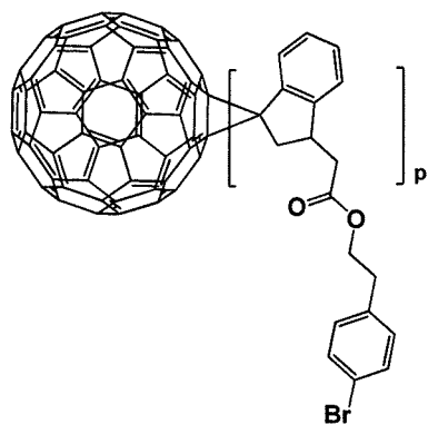
[Formula 1-1-23]
