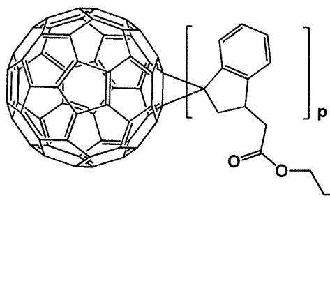
[Formula 1-1-19]
