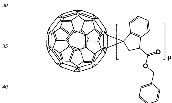
[Formula 1-1-5]
