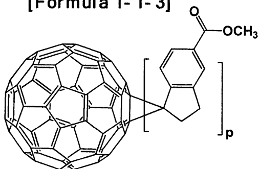
[Formula 1-1-3]
