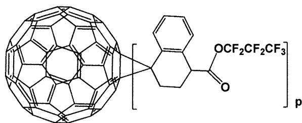
[Formula 1-1-8]
