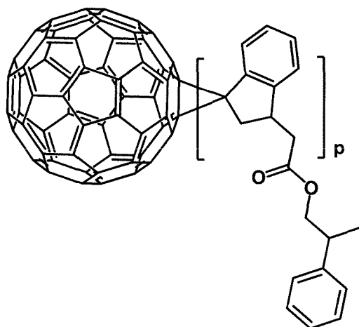
[Formula 1-1-43]
