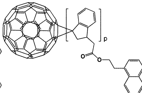
[Formula 1-1-18]
