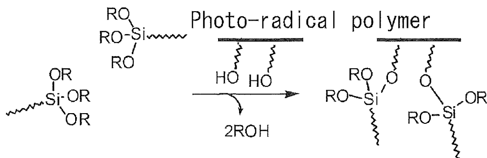
[Chemical 3]
