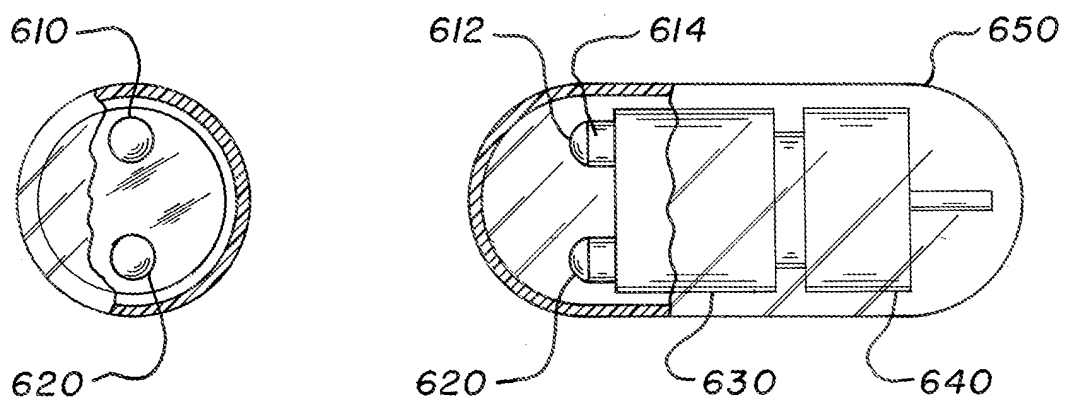
FIG. 6 600
