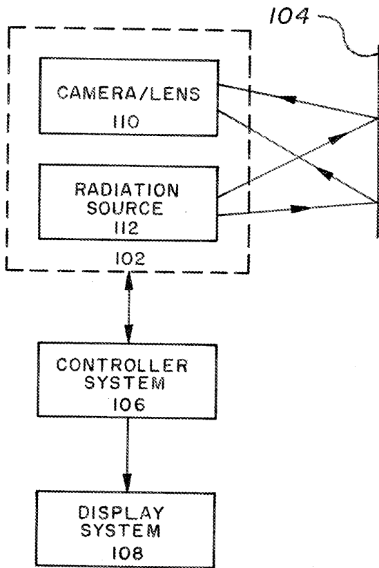
FIG. 1 100
