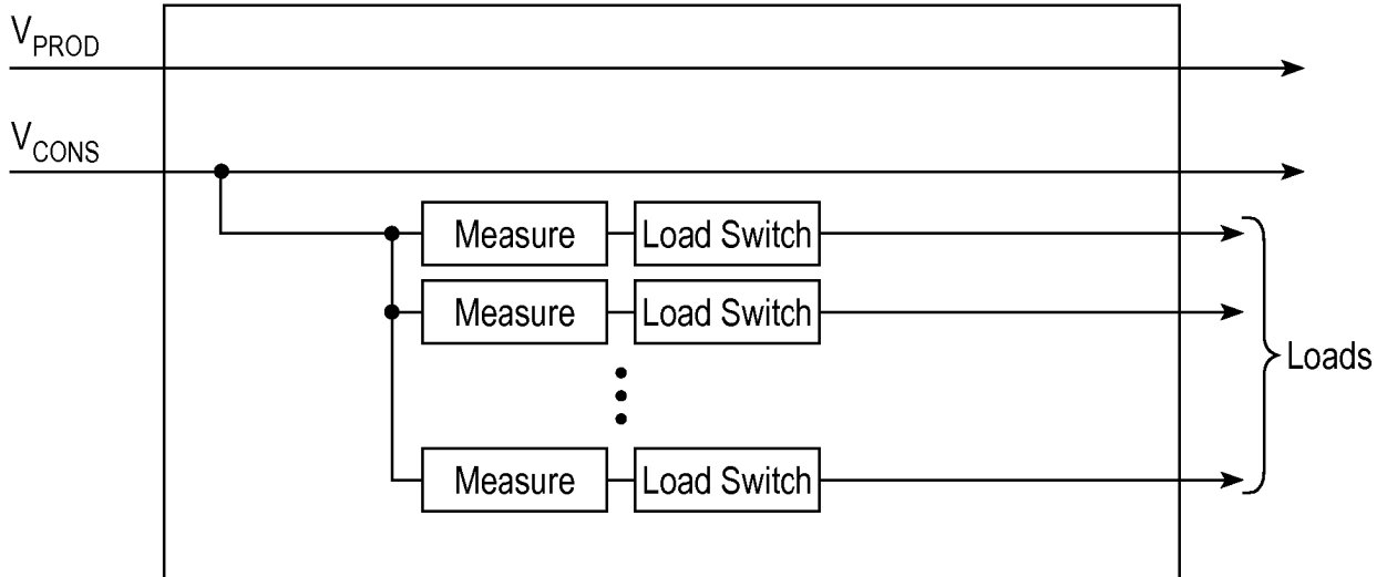
FIG. 15 – Load Switch Module
