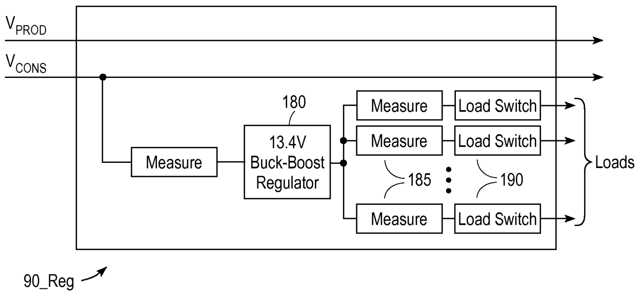
FIG. 14 – 13.4V Regulator Module
