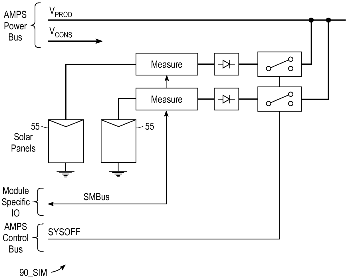
FIG. 13 – Solar Input Module
